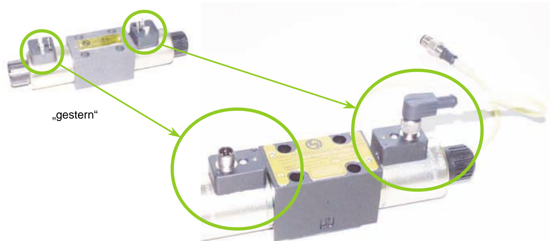
Wegeventil mit M12 x 1-Anschluss nach DESINA
